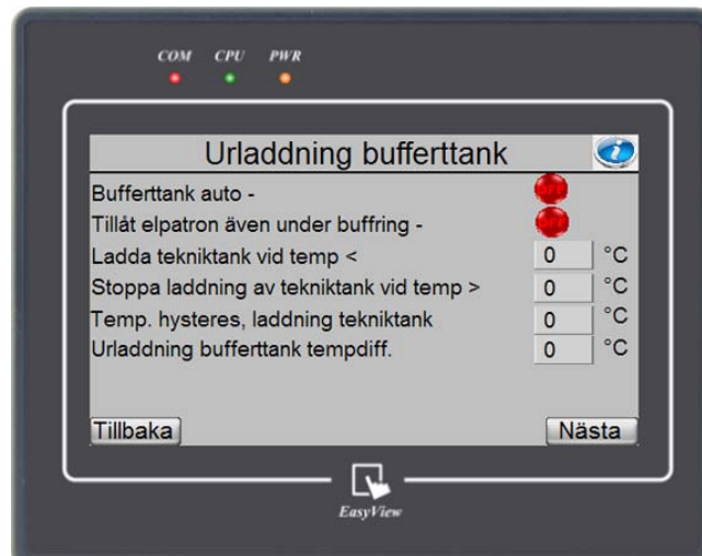
Figur 7. Meny "Urladdning bufferttank"
