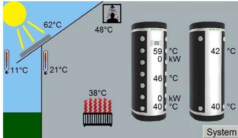
Figur 1. Startmeny systemtank och buffertank
